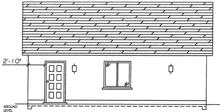
RIGHT ELEVATION
